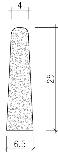
a-a kesiti
