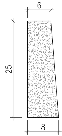
b-b kesiti
