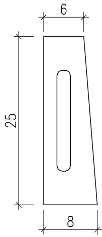
a-a görünüşü
