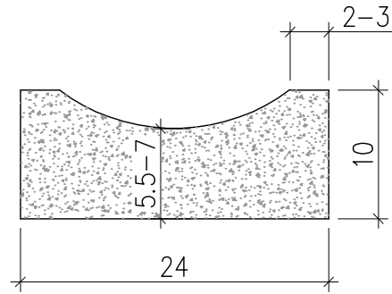
a-a kesiti
