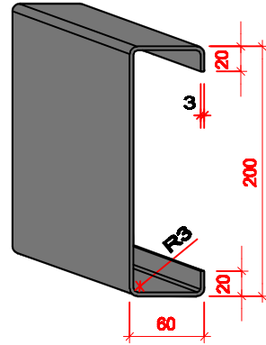
C200.60.3
