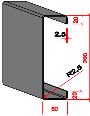
C200.60.2.5
