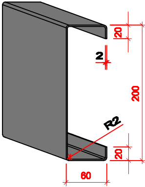
C200.60.2
