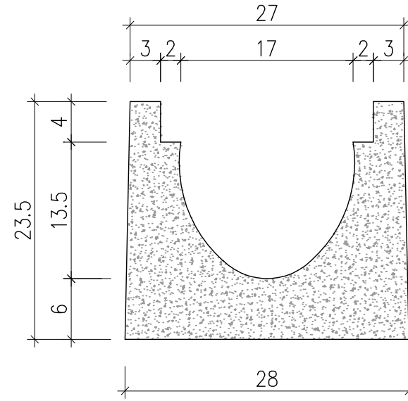
b-b kesiti
