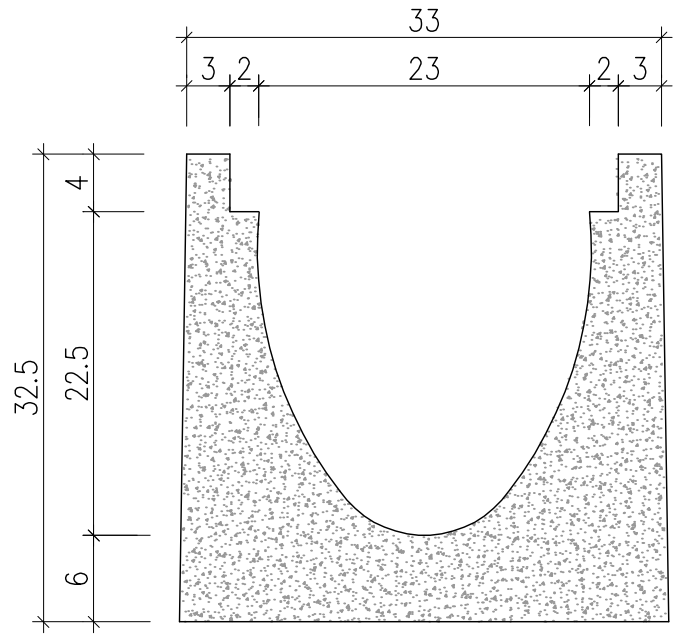
b-b kesiti
