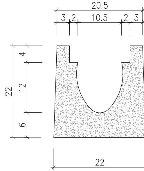
b-b kesiti
