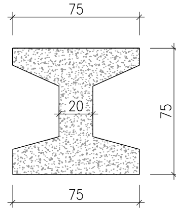
a-a kesiti
