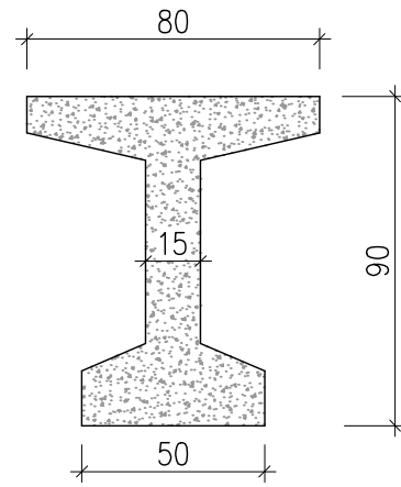
a-a kesiti
