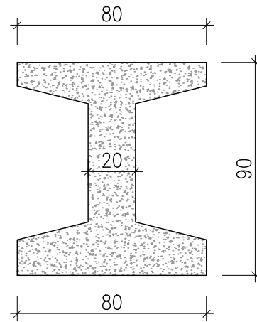
a-a kesiti
